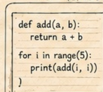
СКРИНШОТЫ ПРОГРАММ
